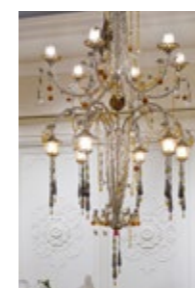
Nome Collezione / Collection Name ARABESQUE Codice Articolo / Article Code CH1352/12AK Misure / Size cm 75X170 N° e Tipo Lampadina / N° & Bulb Type N° 12 Max 28 Watt G9
